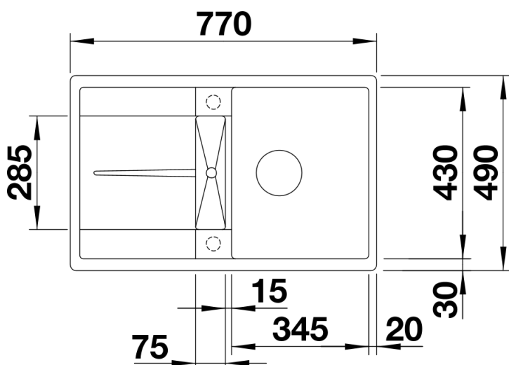
Aufsicht
