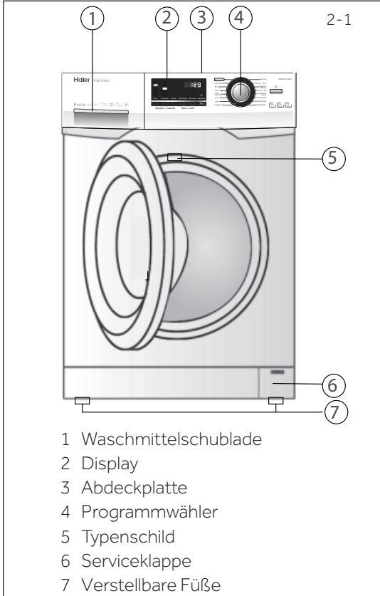
Gerätevorderseite (Abb. 2-1):
