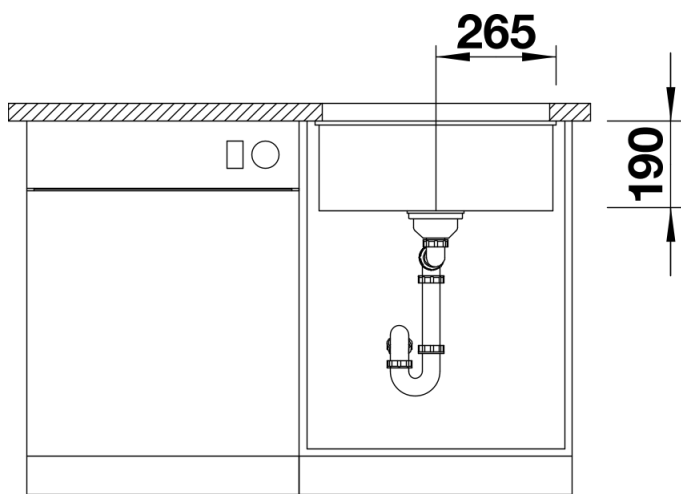
Frontansicht
