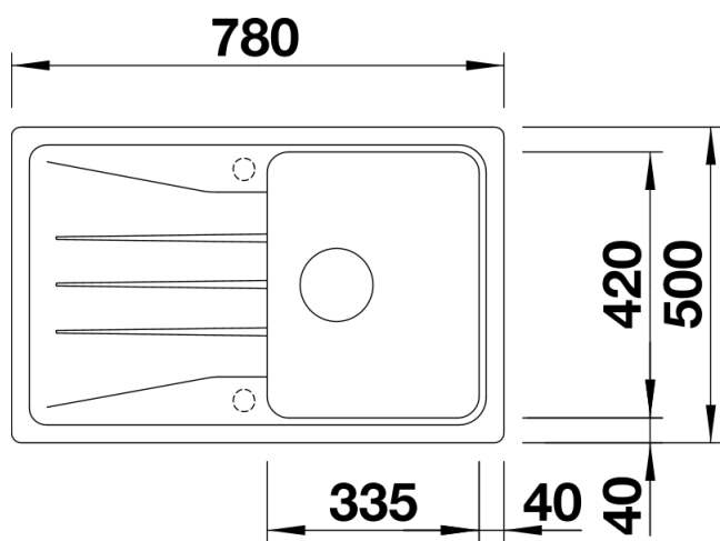
Aufsicht
