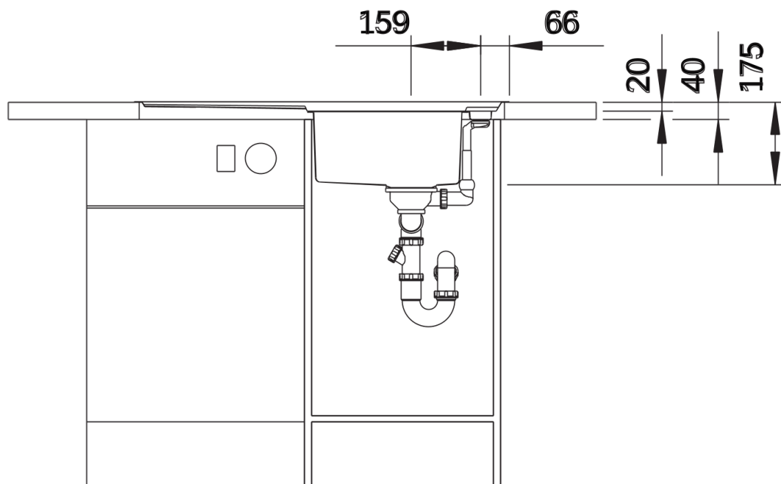
Frontansicht
