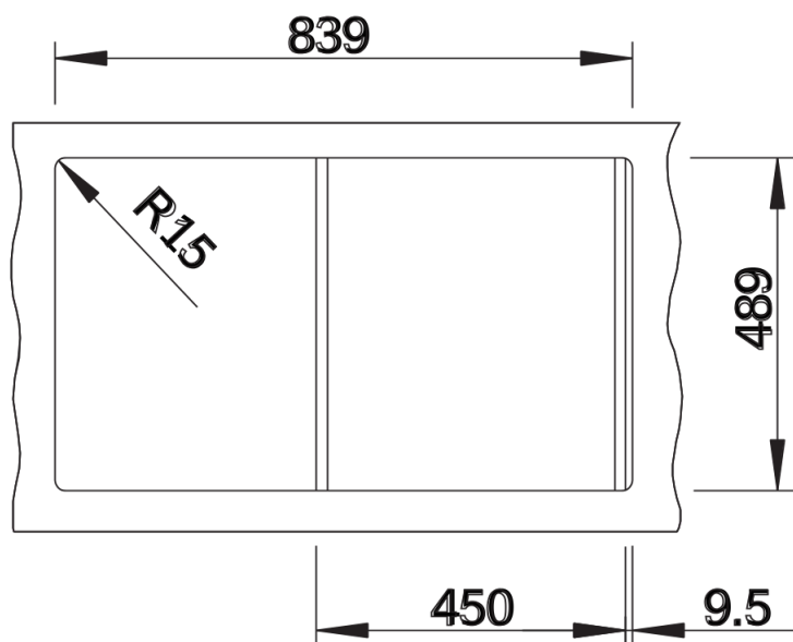
Ausschnitt
