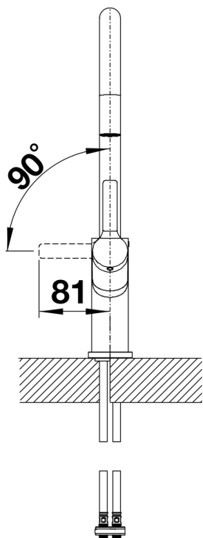
Seitenansicht Hebel 2D
